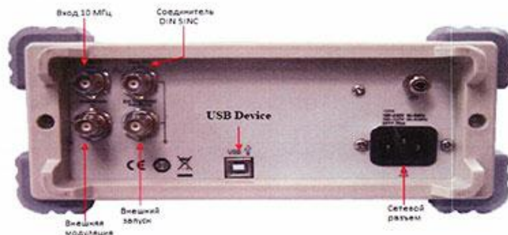
Рисунок 2 – Вид задней панели вольтметра
