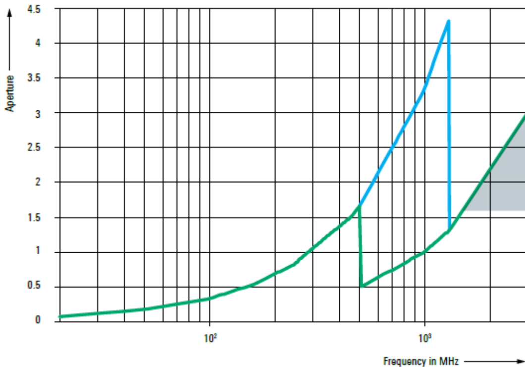
Рис. 4-2. Сравнение аперттуры типовых пятиэлементных систем (зеленый) и пеленгаторных антенн производства Rohde & Schwarz (синий)
