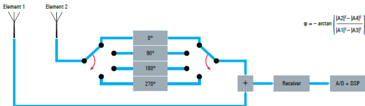
Рис. 4-1. Метод корреляционного интерферометра
