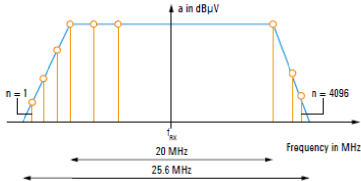
Рис. 1-15. Построение спектра ПЧ
