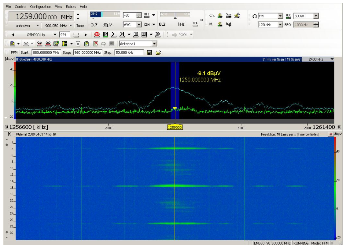
Рис. 1-12. Спектр и временная диаграмма излучения радара
