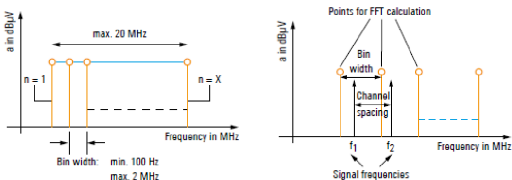
Рис. 1-18. Разрешение сигнала в режиме панорамного сканирования (слева). Соответствие ширины частотного бина ширине канала (справа)
