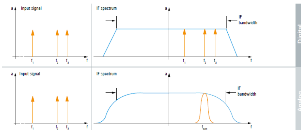
Рис. 1-16. Цифровой (сверху) и аналоговый (снизу) механизм обработки сигналов
