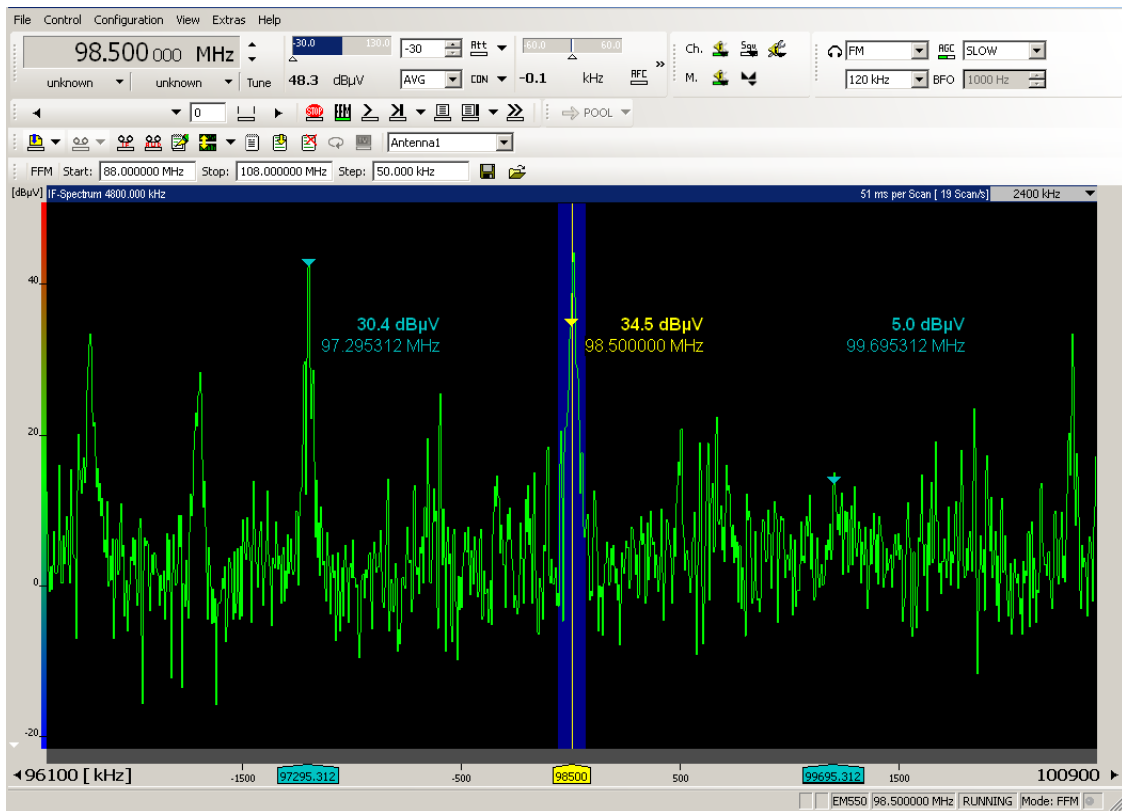
Рис. 1-11. Спектр ПЧ и маркерные функции
