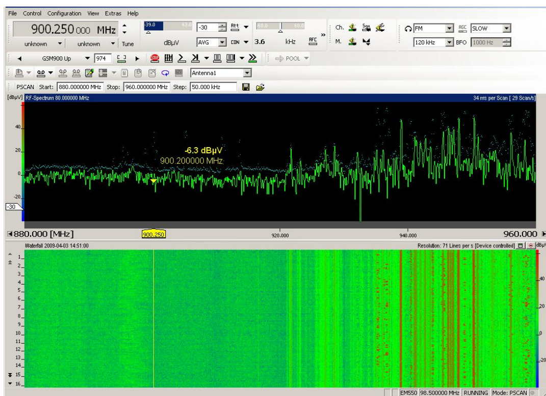
Рис. 1-10. Панорамное сканирование и режим временной диаграммы
