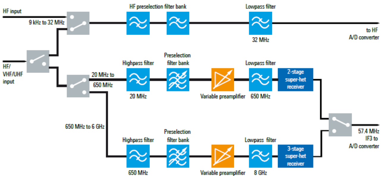
Рис. 1-13. Блок-диаграмма входных каскадов
