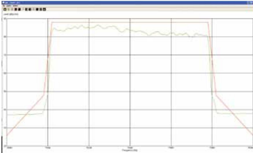
Рис. 1-7. Сравнение спектров DVB-T передатчика
