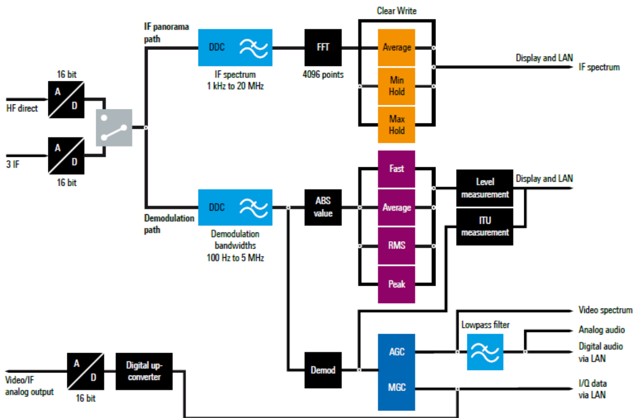
Рис. 1-14. Блок-схема обработки сигналов
