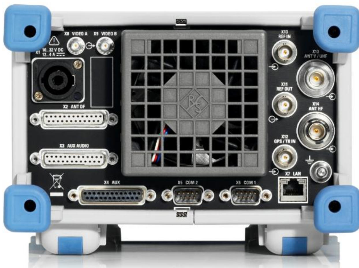
Рис. 1-1. R&S®EB500, вид сзади.
