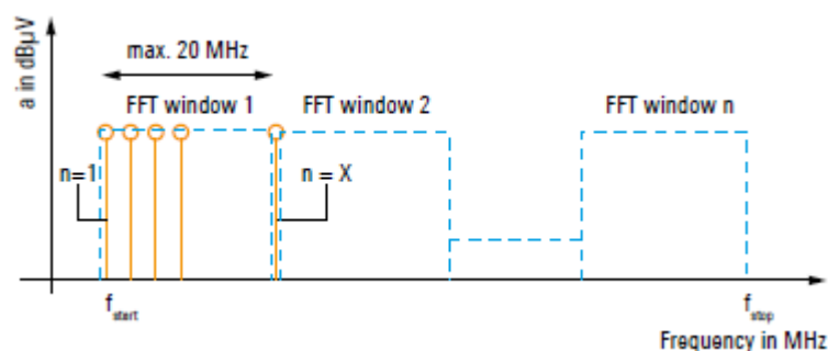
Рис. 1-17. Механизм обработки сигналов в режиме панорамного сканирования
