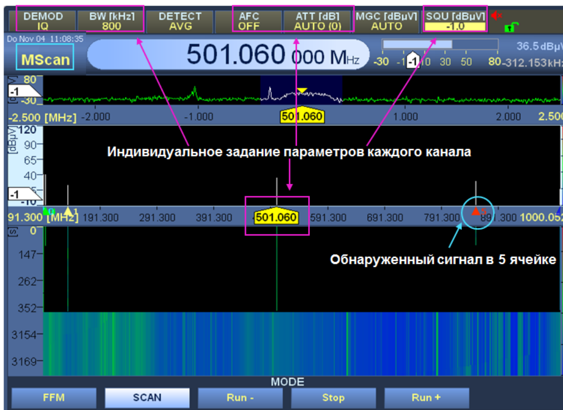
Рис. 1-6. R&S®EB500. Функция сканирования по памяти
