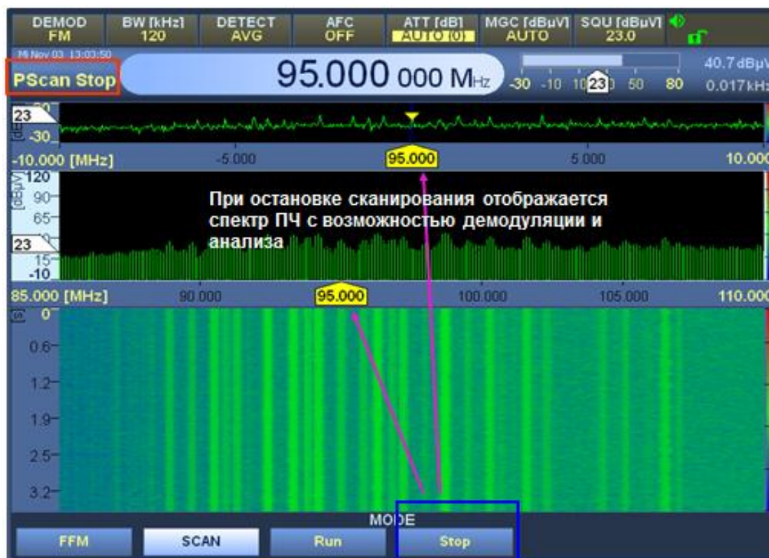
Рис. 1-2. R&S®EB500. Режим панорамного сканирования
