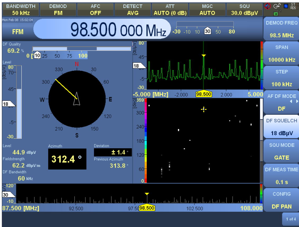
Рис. 1-4. R&S® EB500. Диаграмма пеленгов
