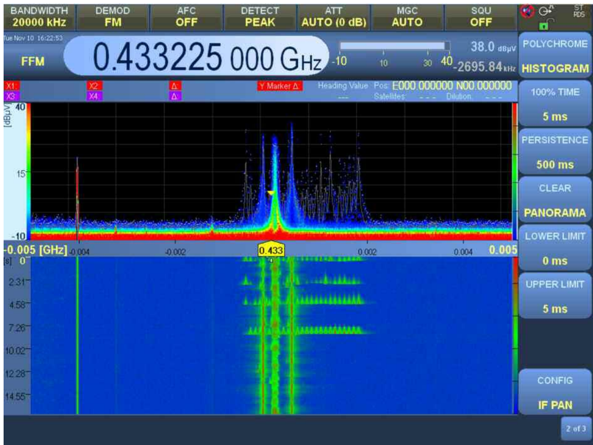
Рис. 1-5. Функция панорамного сканирования
